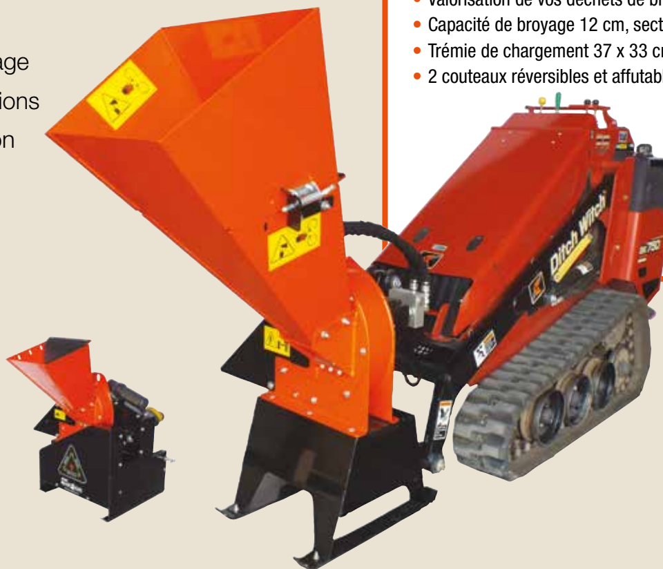
Broyeur adaptable sur robot télécommandé.
